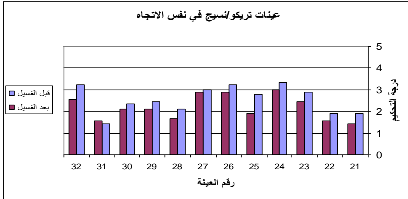
شكل (٩) متوسطات درجات التحكيم لعينات تريكو / نسيج قبل وبعد الغسيل في نفس الاتجاه
