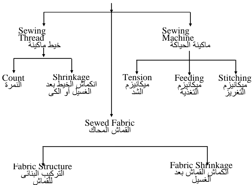
شكل (١) يوضح تأثير عناصر الحياكات الثلاثة في كرمشه الوصلات
