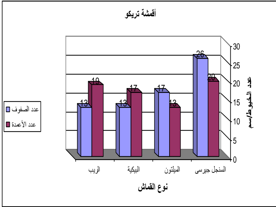
شكل (٥) عدد الصفوف والأعمدة لعينات قماش التريكو /سم
