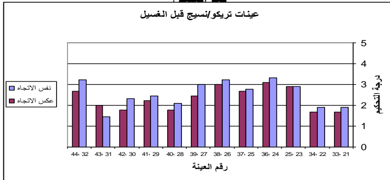
شكل (١٥) متوسطات درجات التحكيم لعينات تريكو / نسيج في نفس وعكس الاتجاه قبل الغسيل
