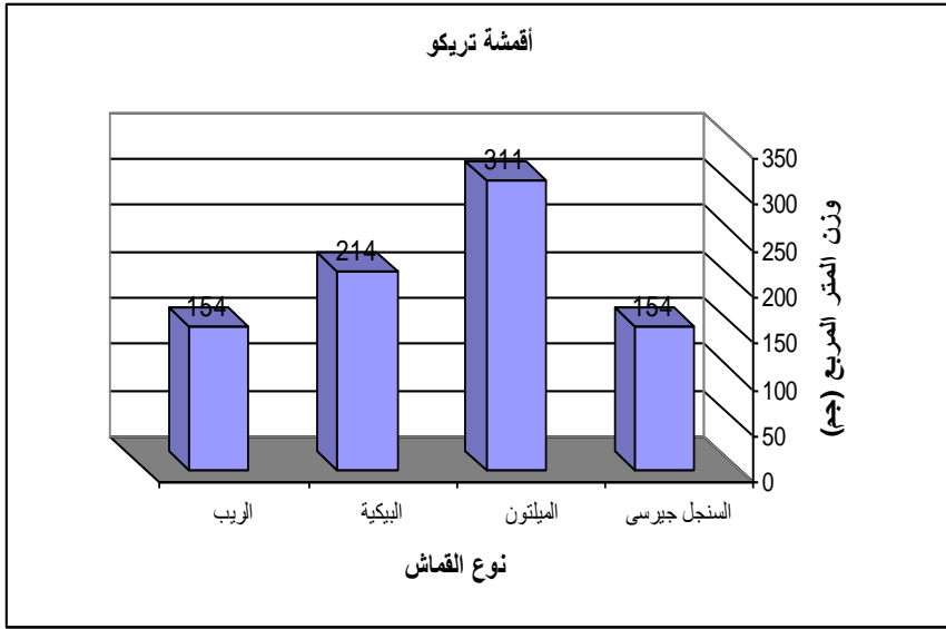
شكل (٣) أوزان عينات قماش التريكو جم/م ٢
