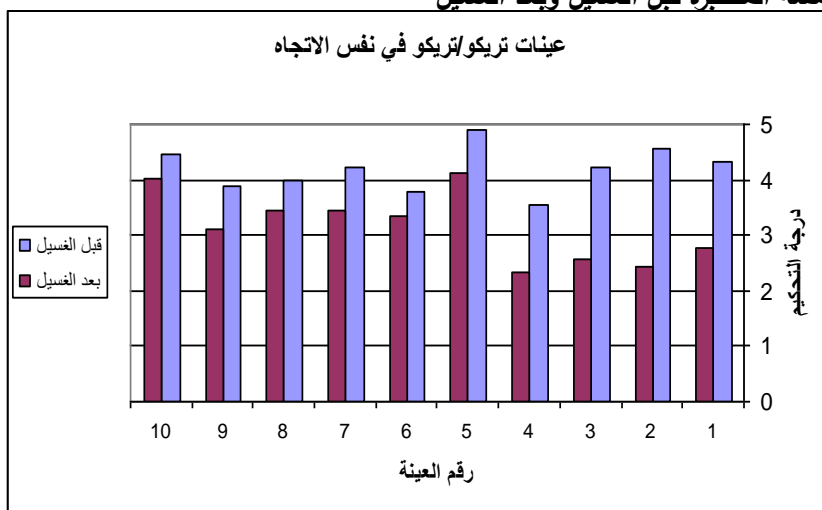
شكل (٧) متوسطات درجات التحكيم لعينات تريكو / تريكو قبل وبعد الغسيل في نفس الاتجاه
