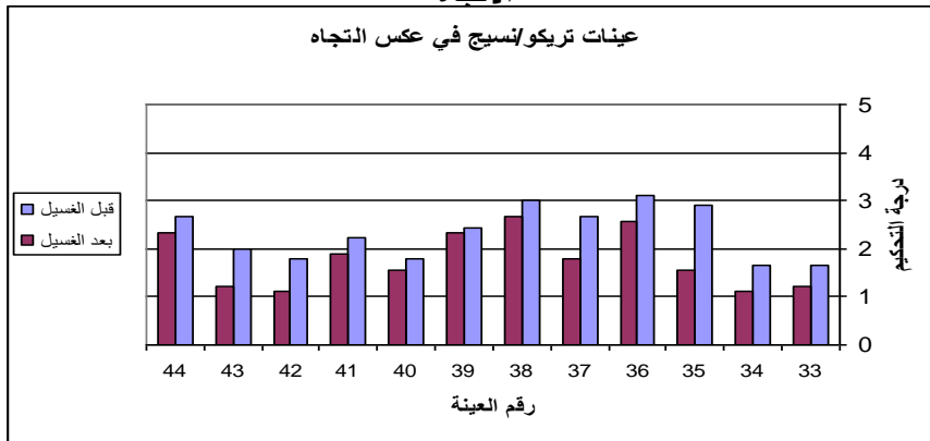
شكل (١٠) متوسطات درجات التحكيم لعينات تريكو / نسيج قبل وبعد الغسيل في عكس الاتجاه
